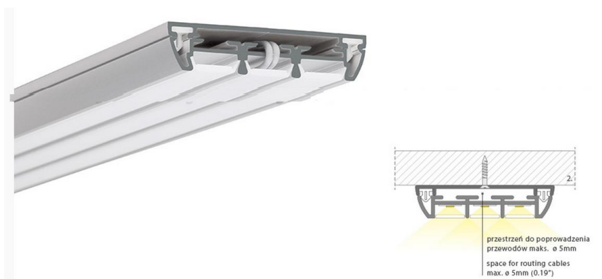
PROFIL TETRA-43
