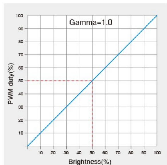
Linear dimming
